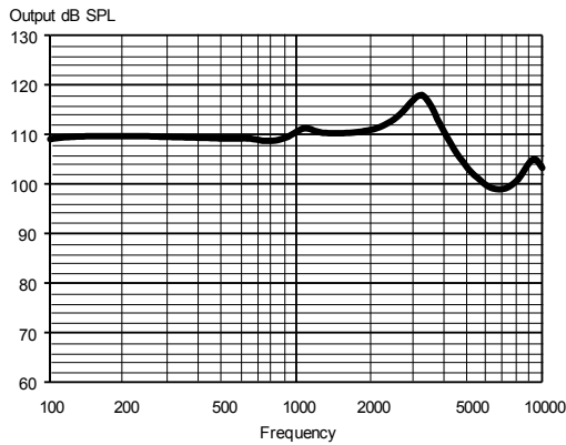
SORTIE MAXIMUM - SIMULATEUR D'OREILLE
