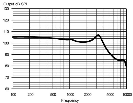
SORTIE MAXIMUM - COUPLEUR 2CC
