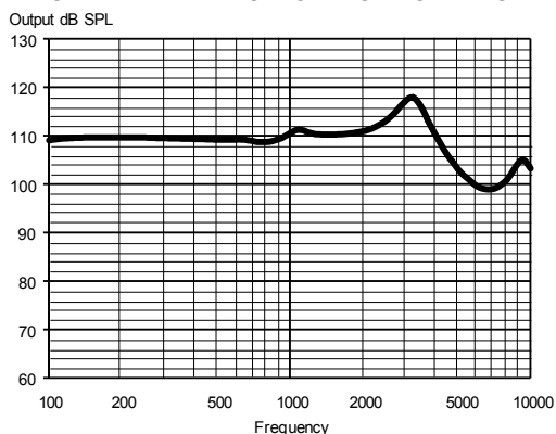
SAÍDA MÁXIMA - SIMULADOR AUDITIVO
