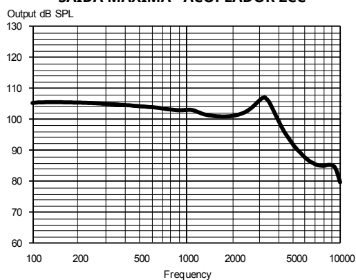
SAÍDA MÁXIMA - ACOPLADOR 2CC
