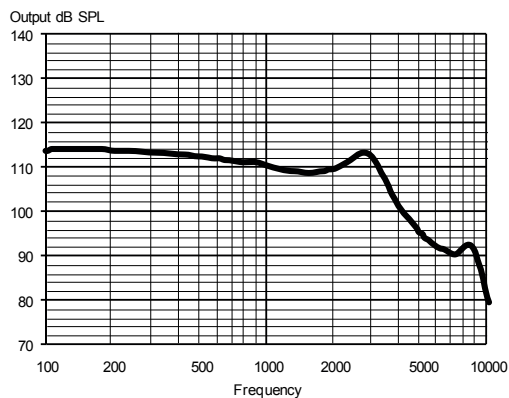
SORTIE - COUPLEUR 2CC
